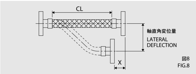
取り付け面間が拘束されず変化できる場合 When the face-to-face distance is not fixed and allowed to change 単位 (mm)
