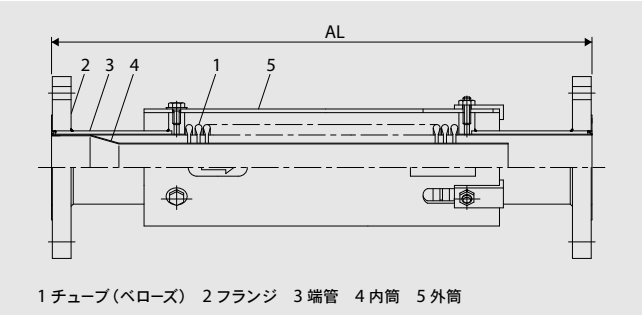
1 チューブ（ベローズ） 2 フランジ 3 端管 4 内筒 5 外筒
