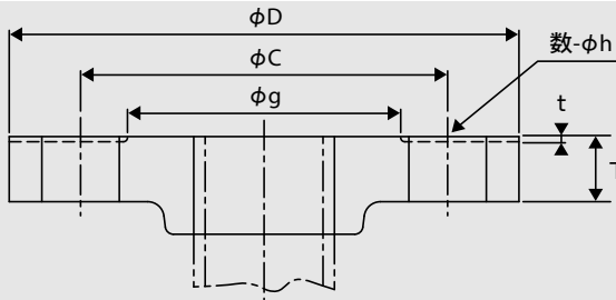
呼び圧力5K フランジの基本寸法(JIS B 2220) BASIC DIMENSIONS OF NOMINAL PRESSURE 5K FLANGE 単位: mm
