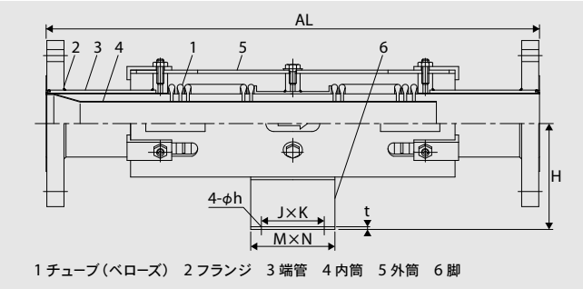
1 チューブ（ベローズ） 2 フランジ 3 端管 4 内筒 5 外筒 6 脚
