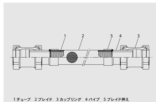
1 チューブ 2 ブレード 3 カップリング 4 パイプ 5 ブレード押え
