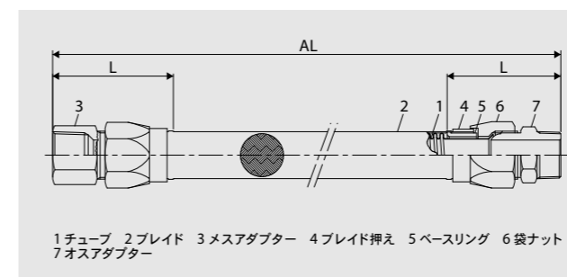
管用テーパ オスアダプター+管用テーパ メスアダプター付 [S215MF]
