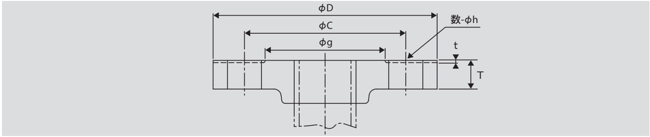
呼び圧力5K フランジの基本寸法(JIS B 2220) BASIC DIMENSIONS OF NOMINAL PRESSURE 5K FLANGE 単位: mm
