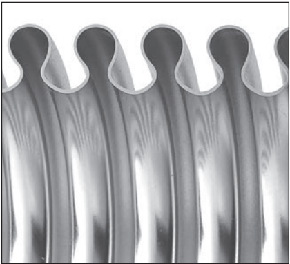
オメガチューブ ANNULAR (OMEGA) PROFILE
