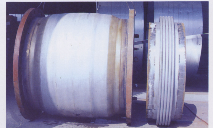
●伸縮実験伸び418mm、縮み215mm 許容量±50mm、破断、漏洩なし、安全性をみごとに立証
