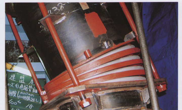
●4倍変位試験 許容値100mm → 400mm 変位させ200回繰返し
