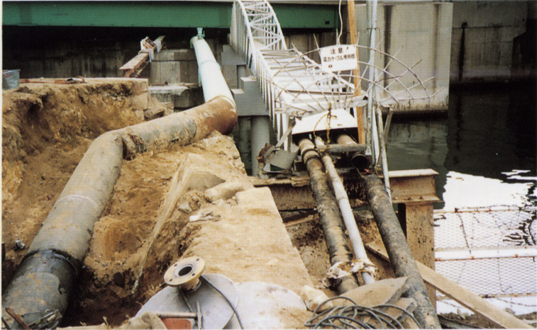
●折れ曲がった水道管、神戸東灘区
