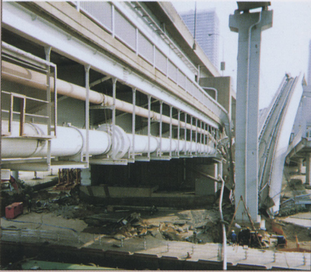
●落下した六甲ライナーの橋桁と異常が見られなかった水道管と伸縮管
