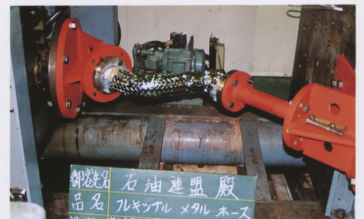
●斜め(45°)の圧縮変位試験 400mm 200 回繰返し
