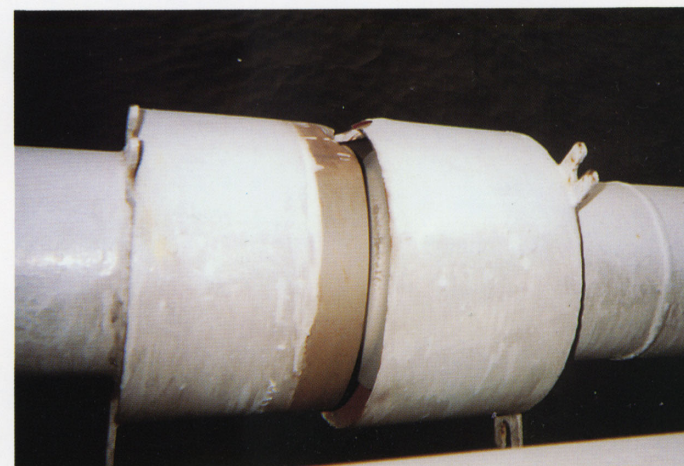
●カバーが抜けて、異常変位したベローズが見える このような変形でも漏水はなく安全性が立証された
